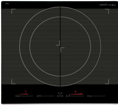
PLACA INDUCCIÓN 60 CM 4 Zonas - 1 Modular Gigante de 40 cm
